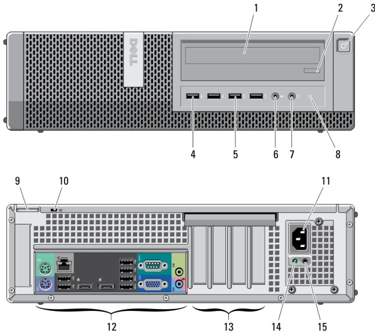
2. ábra. Asztali kivitel elő- és hátulnézete
